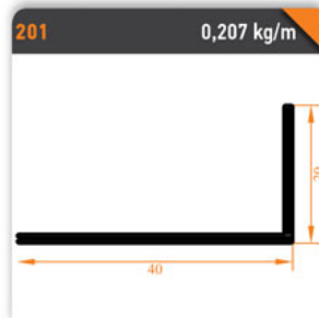
20x40 Köşebent 20x40 Bracket
