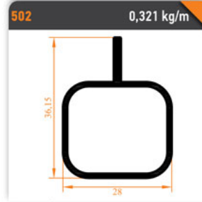
Çamaşırılık Borusu Laundry Hanger Tube
